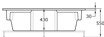
Alzado
