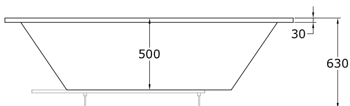
Alzado
