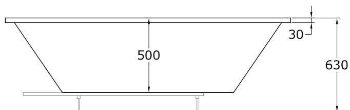
Alzado
