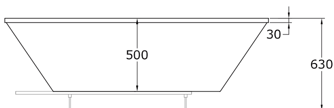
Alzado
