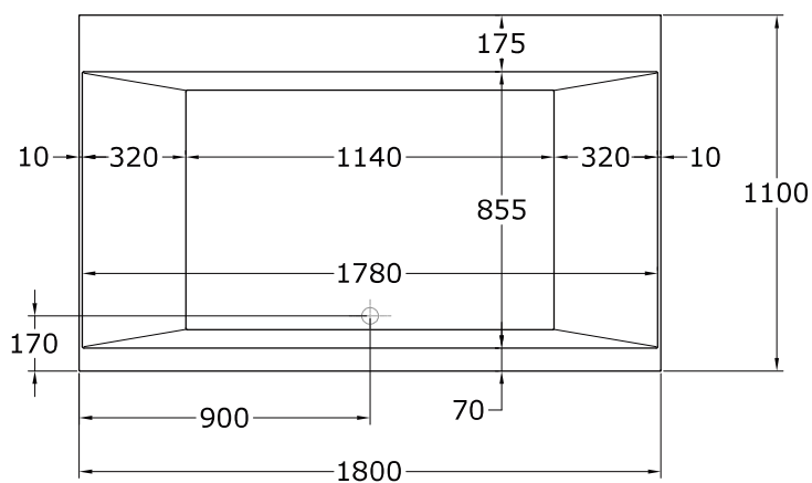
Planta
