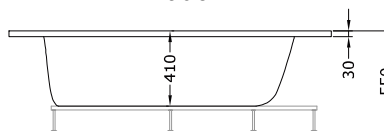
Alzado
