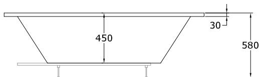
Alzado
