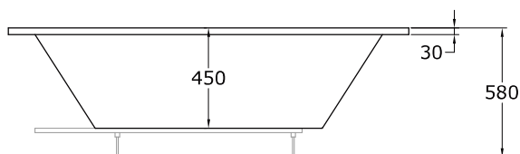
Alzado
