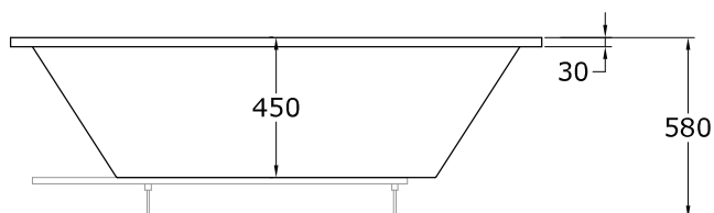
Alzado
