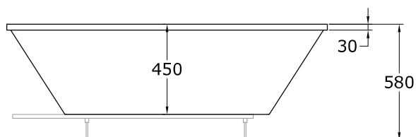
Alzado
