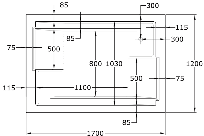
Planta
