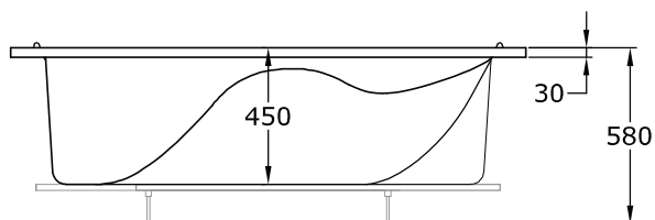
Alzado
