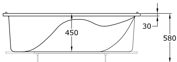
Alzado
