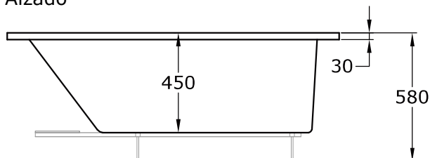
Alzado
