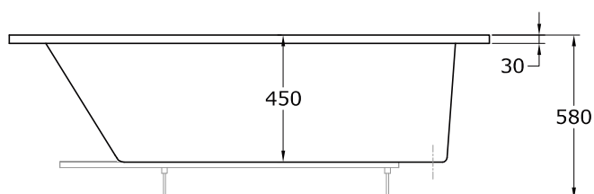
Alzado
